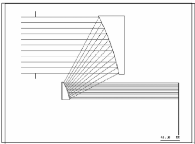
图 3 光学系统图
