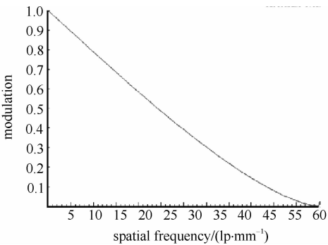
图 4 调制传递函数曲线
