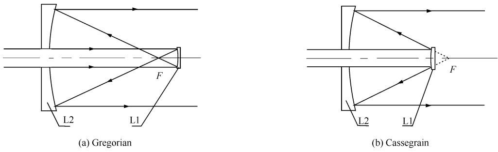
图 2 无焦格里格利和焦卡塞格林扩束系统
